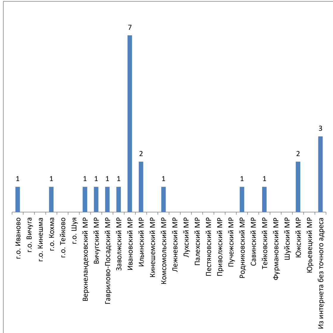
География обращений
